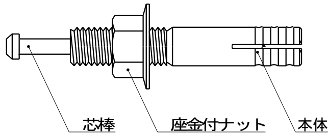
ハイアンカー PCタイプの部品構成
