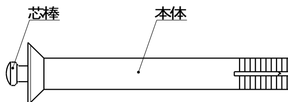
ハイアンカー SYタイプの部品構成
