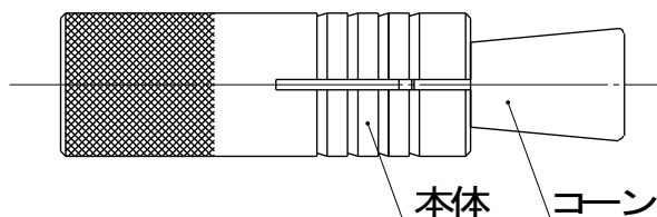
ハイアンカー SNタイプの部品構成
