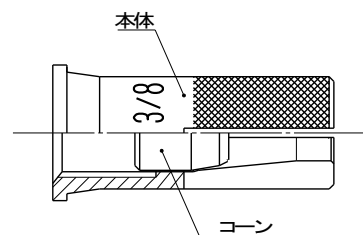
ハイアンカーSTNW3030 の 部品構成
