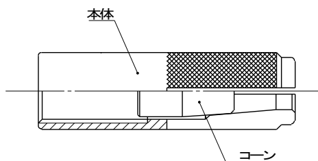
ハイアンカーSTN タイプ(STNW3030 除く)の 部品構成
