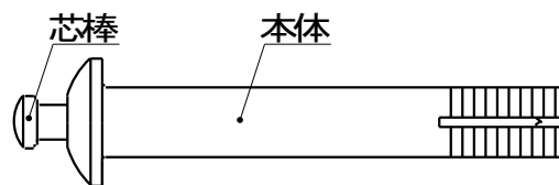
ハイアンカー PT タイプの部品構成
